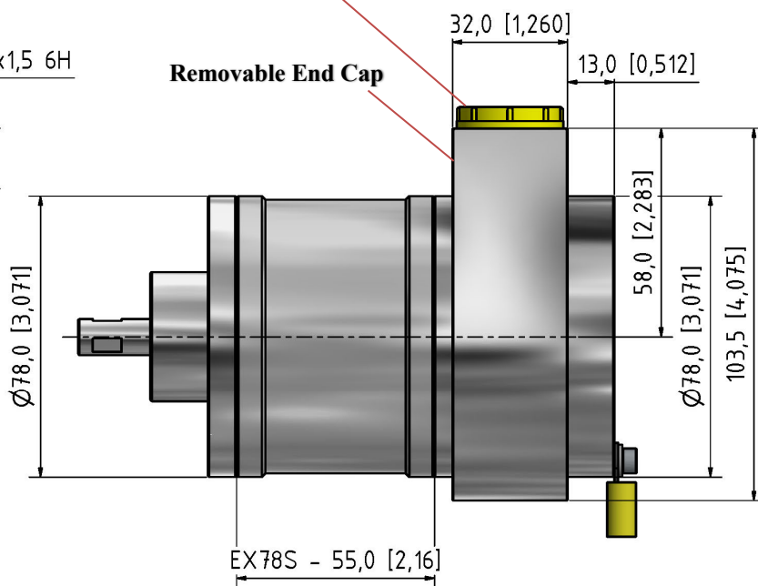
Side M25 End Cap (FI)
