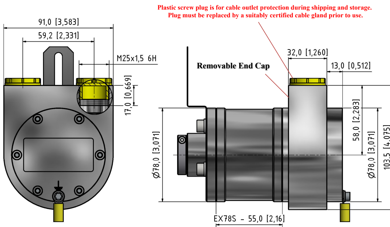
Side M25 End Cap (FI)
